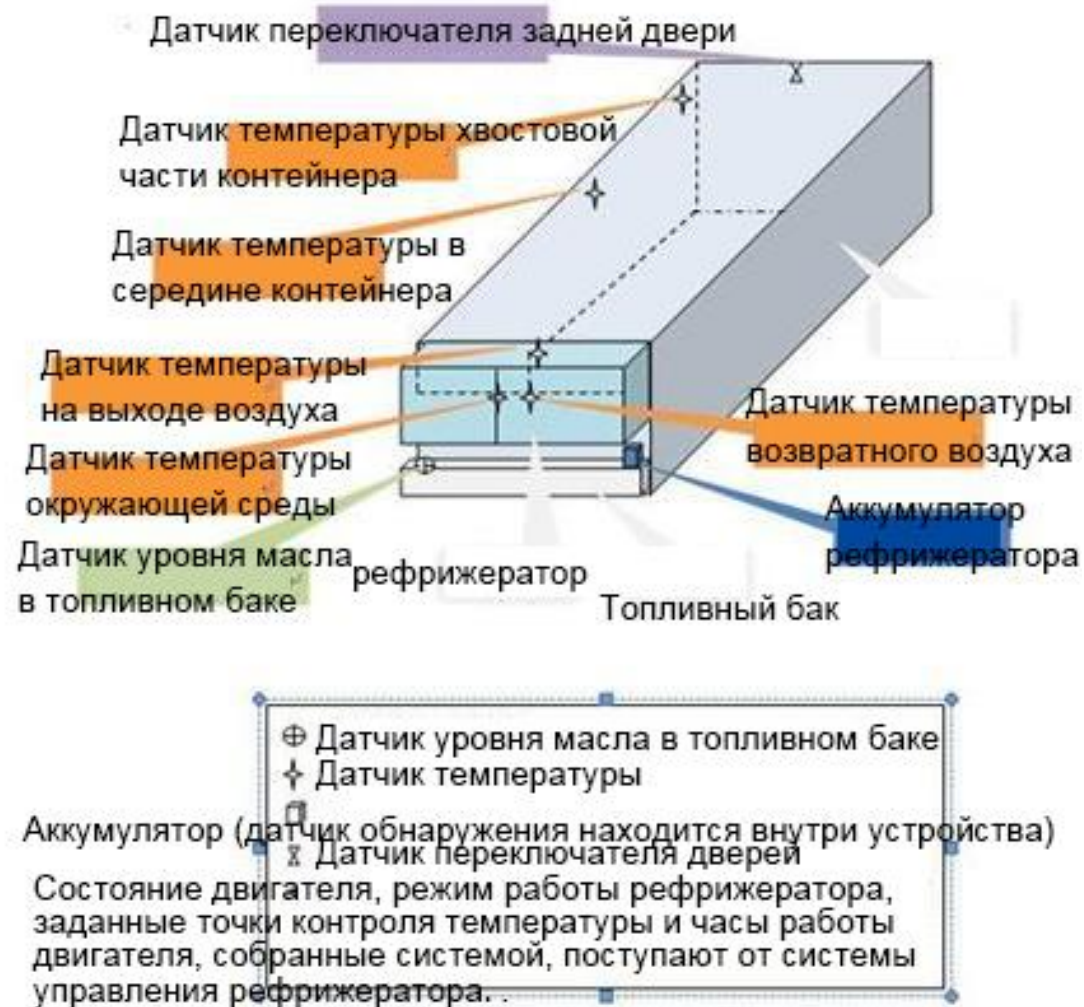
Принципиальная схема датчика рефрижераторных контейнеров
